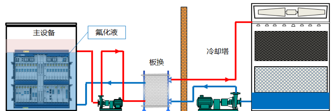
图 9 浸没液冷+冷塔散热架构示意图
