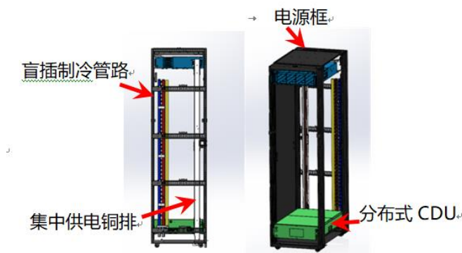
图 8 盲插解耦方案
