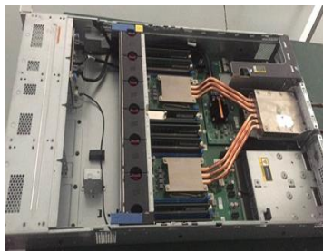
图2 中国移动呼和浩特冷板式液冷测试
