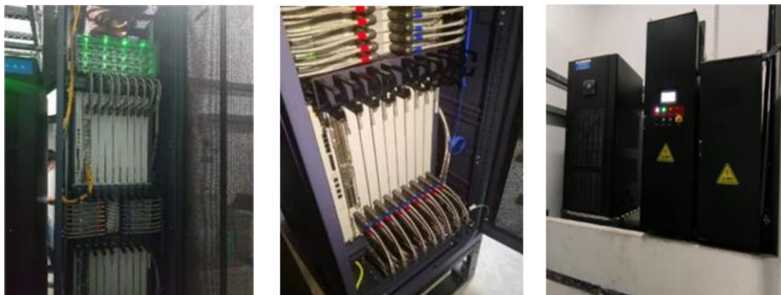
图 5 中国电信贵州冷板式液冷路由器试点
