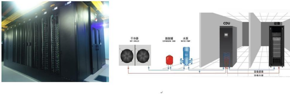
图 7 中国电信广州数据中心冷板式液冷微模块试点
