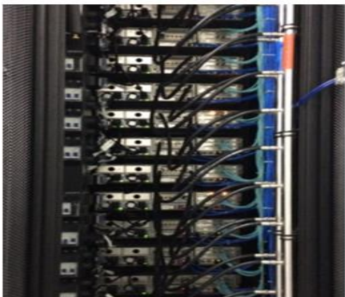
图1 中国移动南方基地气液双通道冷板液冷研究和实践
